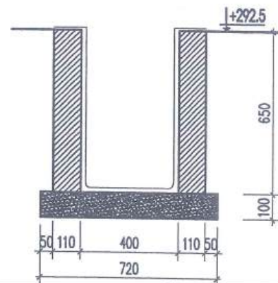
MẶT CẮT RÃNH HỖ H2-H3 TẠI H2
