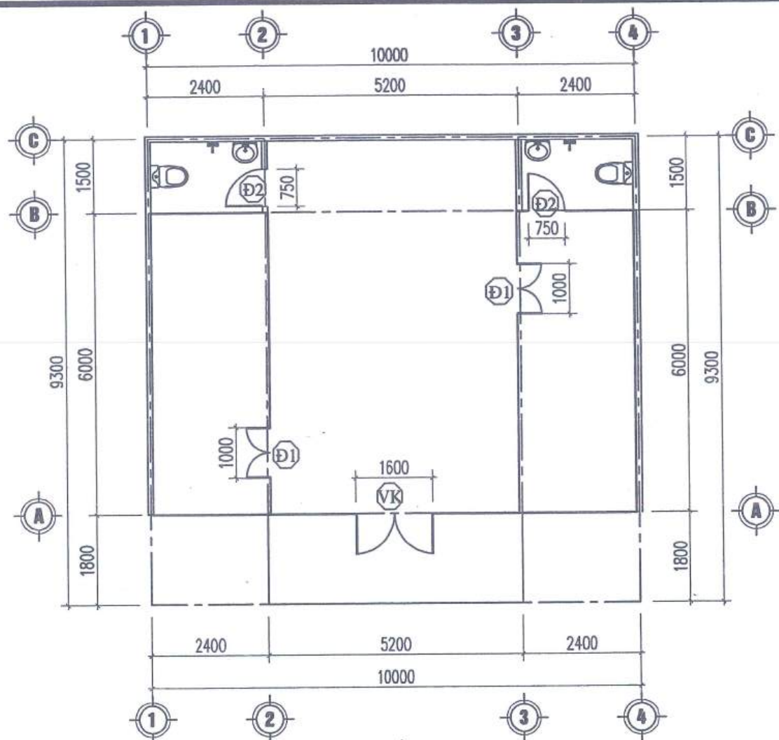
MẶT BẰNG
