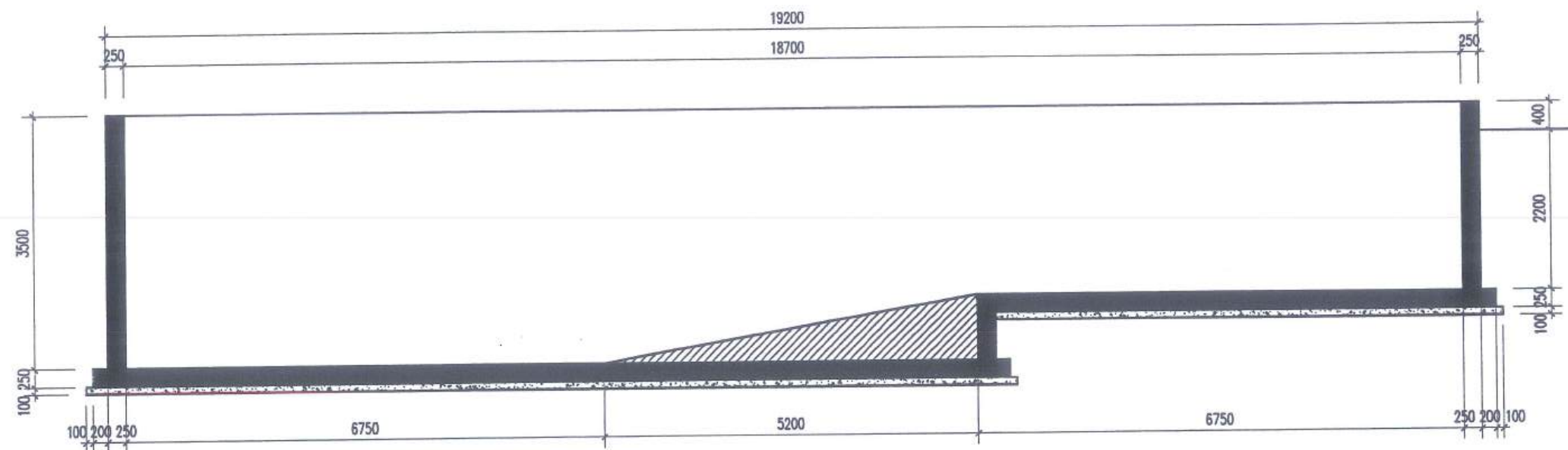
CẮT A-A
