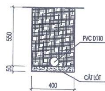
MẶT CẮT RĂNG ĐẶT ỐNG THOÁT NƯỚC THẢI SÂN XUẤT
