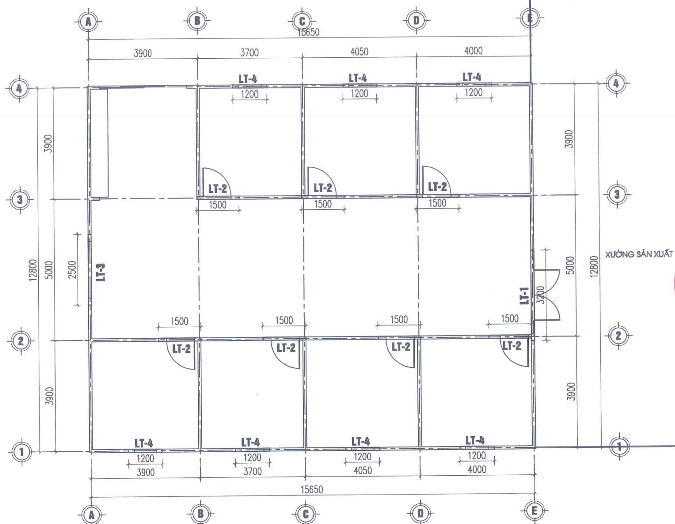
MẶT BẰNG LANH TÔ
