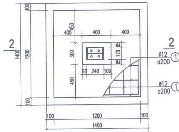
MÓNG M-2 (SL: 04)
