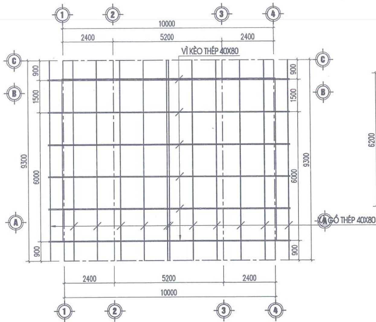
MẶT BẰNG MÁI VÌ KÈO XÀ GỖ MÁI
