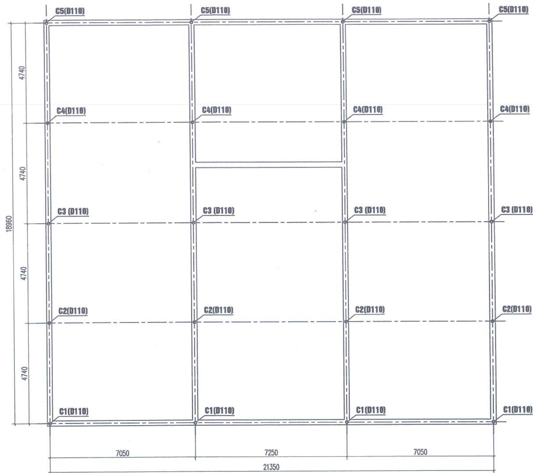
MẶT BẰNG
