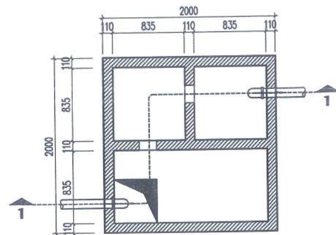
MẶT BẰNG BỂ TỰ HOẠI
