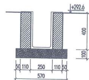
MẶT CẮT RĂNG ĐẶT ỐNG THOÁT NƯỚC THẢI SÂN XUẤT
