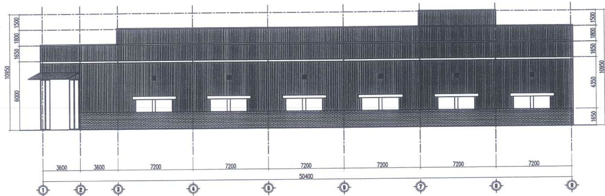
MẶT ĐỨNG TRỤC 1-9
