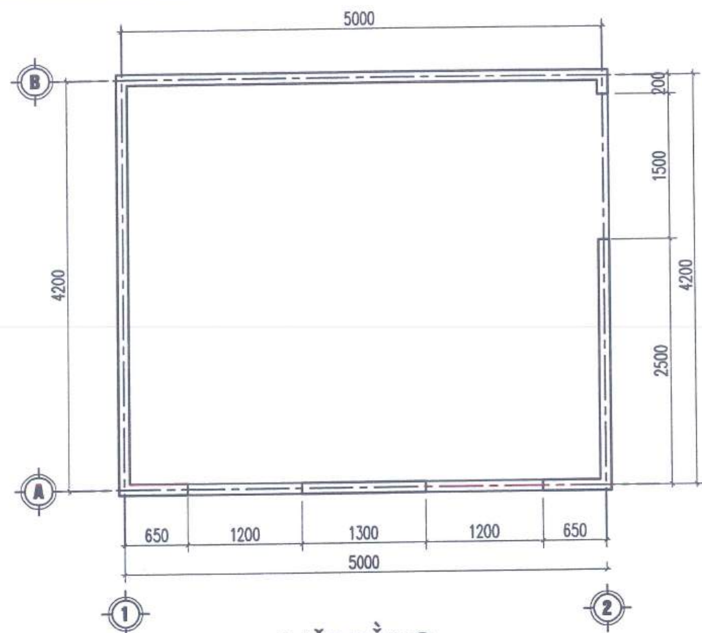
MẶT BẰNG
