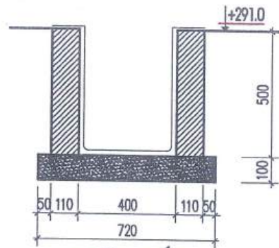
MẶT CẮT RÃNH HỖ H4-H5 TẠI H4
