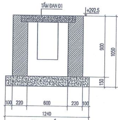
MẶT CẮT HỖ GA H2
