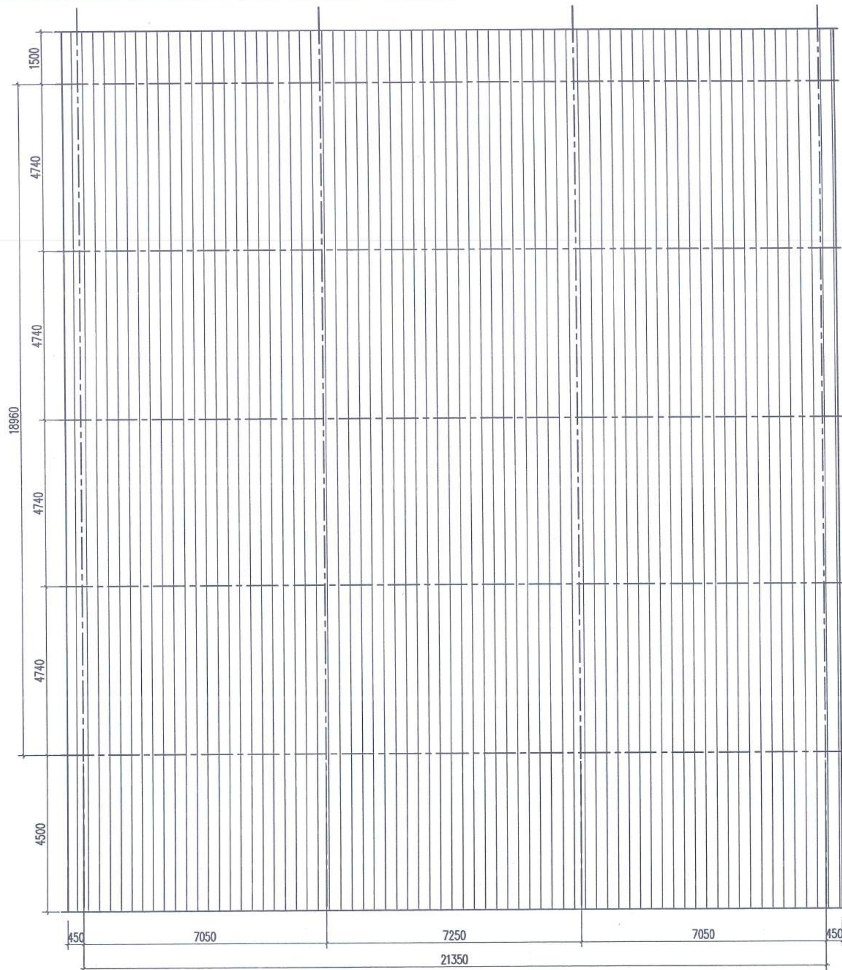
MẶT BẰNG MÁI TÔN
