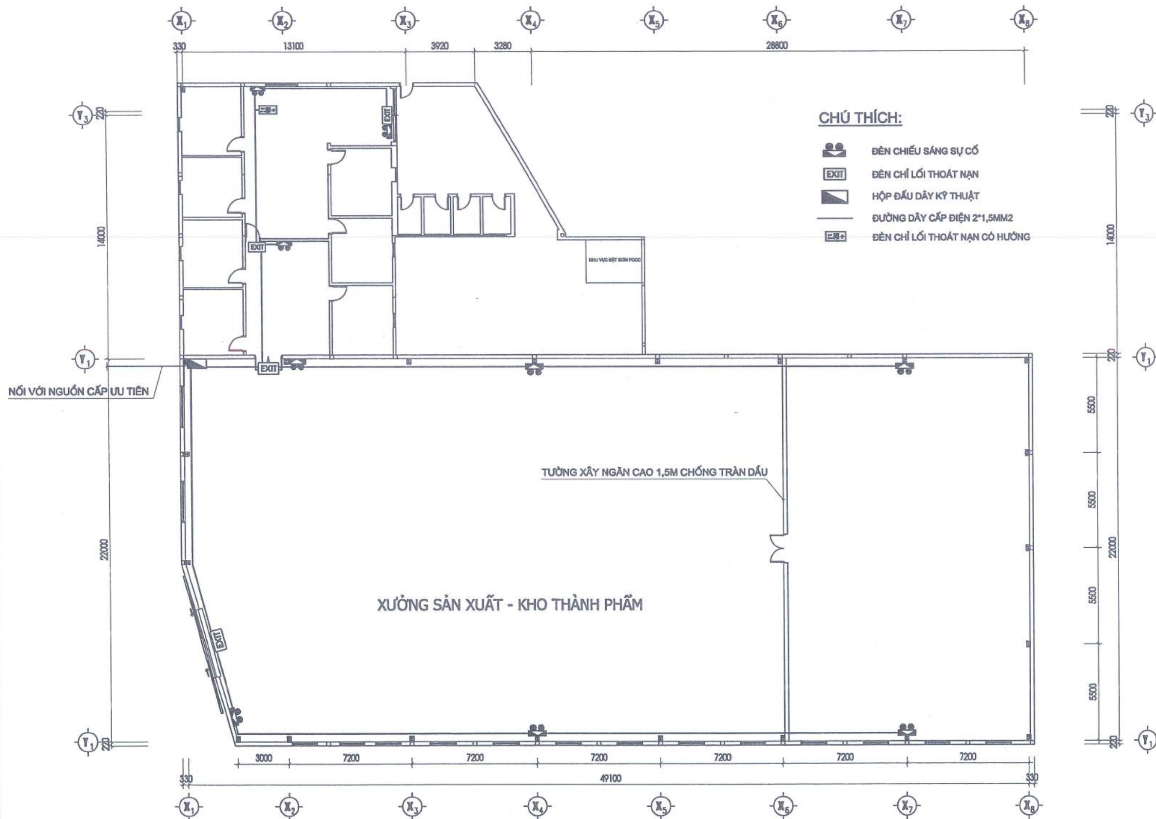
MẶT BẰNG HỆ THỐNG ĐÈN CHIẾU SÁNG SỰ CỐ, ĐÈN EXIT THOÁT NẠN XUỒNG SẢN XUẤT - KHO THÀNH PHẨM
