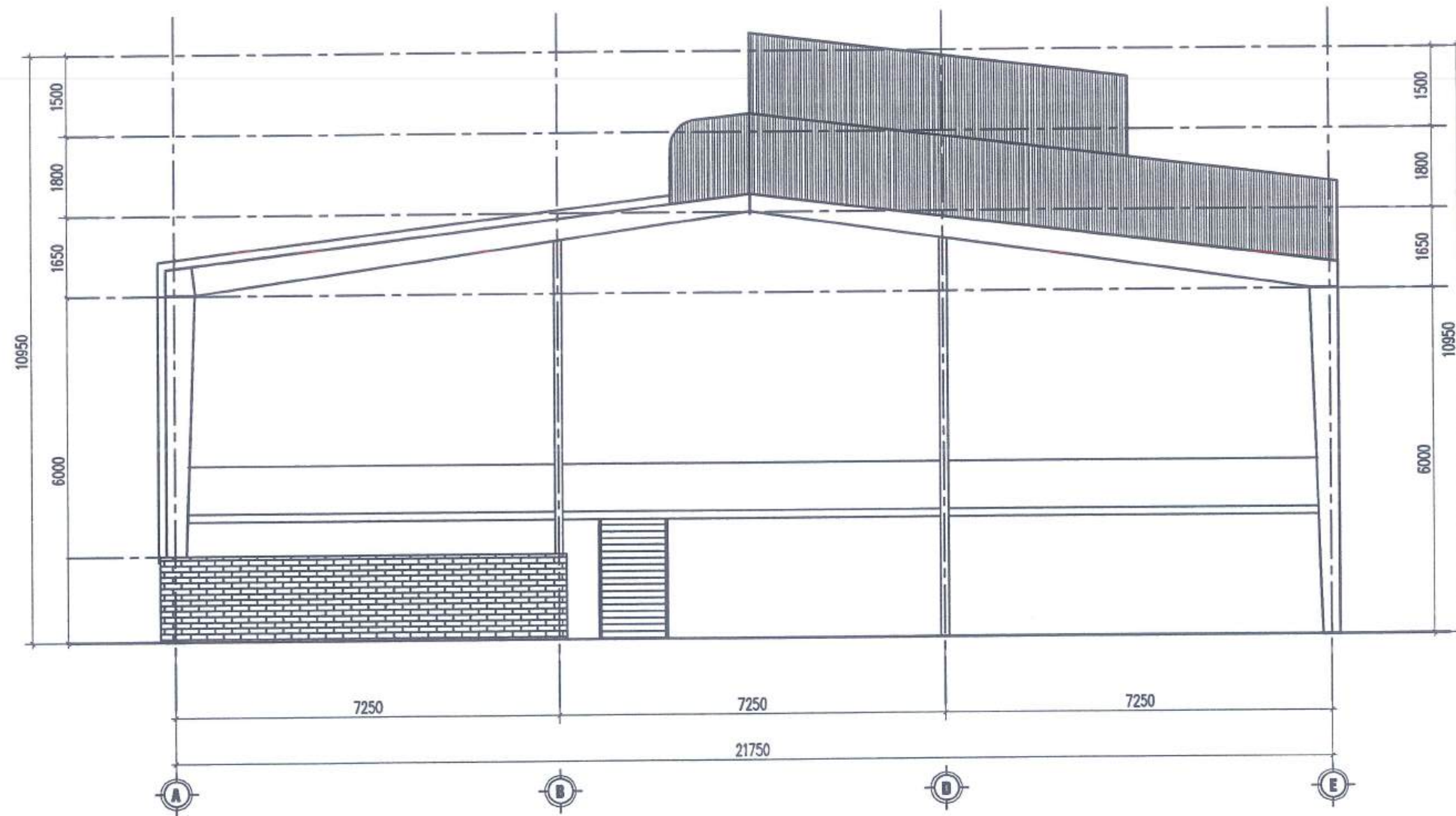
MẶT ĐỨNG TRỤC A-E
