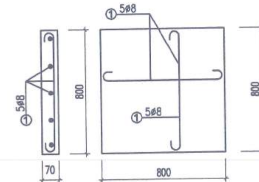
CỐT THÉP ĐÀN NẮP BỂ
