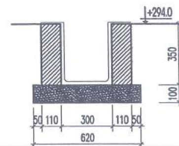
MẶT CẮT RÃNH HỖ R2-H1 TẠI R2
