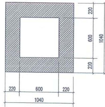
MẶT BẰNG HỖ GA H1, H2, H3, H4
