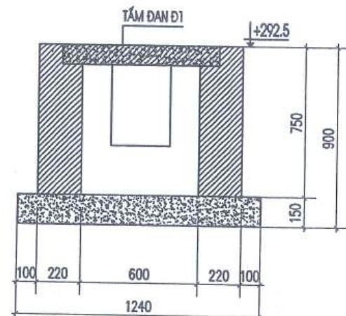
MẶT CẮT HỖ GA H1
