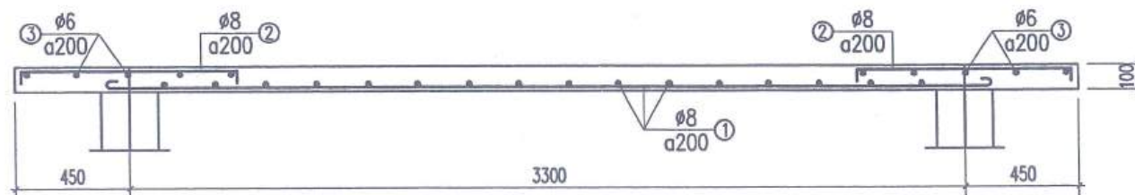
MẶT CẮT CỐT THÉP MÁI
