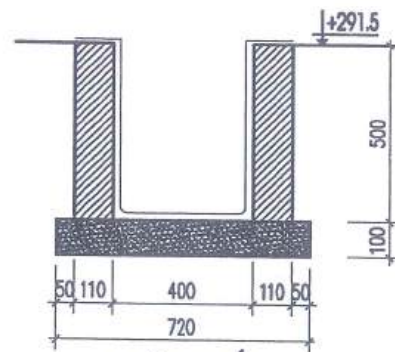
MẶT CẮT RÃNH HỖ H2-H3 TẠI H3
