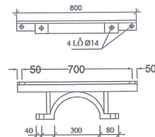
CHI TIẾT 6
