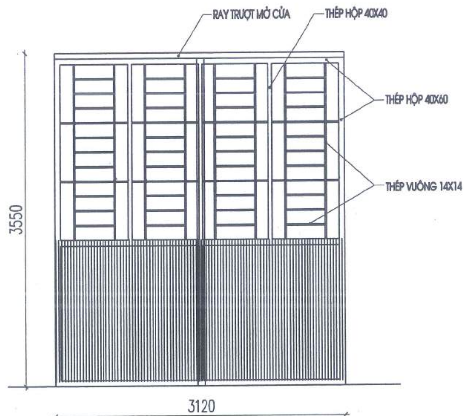
CỬA Đ1 (CỬA THÉP)
