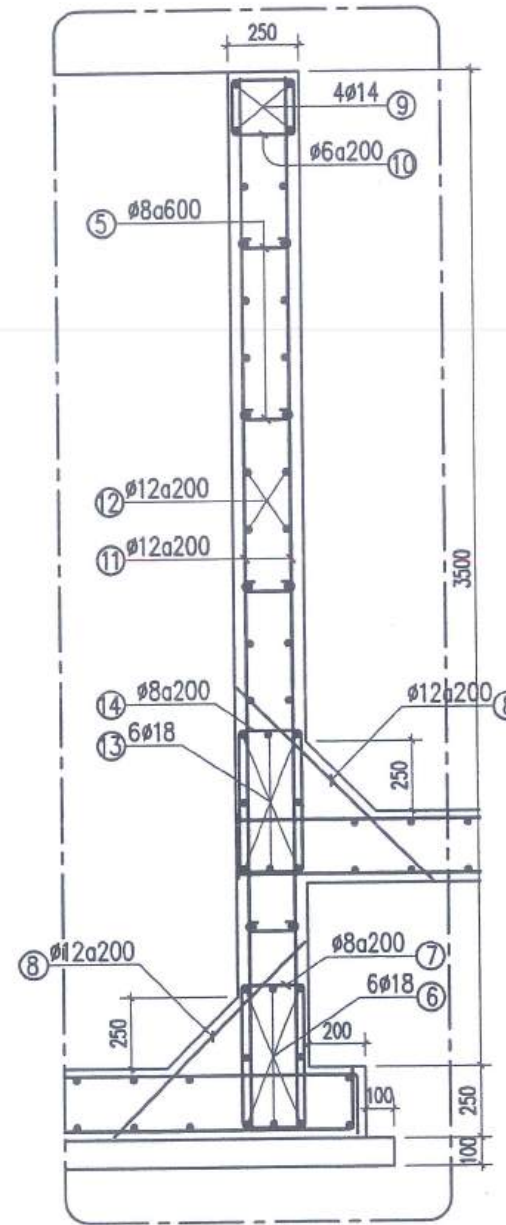
CẮT 3-3
