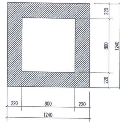
MẶT BẰNG HỖ GA H5
