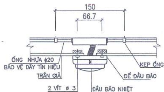
LẮP ĐẶT ĐẦU BÁO KHỎI QUANG HỌC DƯỚI XÀ THÉP
