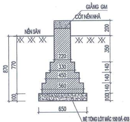
MÓNG MG-1
