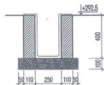
MẶT CẮT RÃNH HỖ R3-H2 TẠI H2
