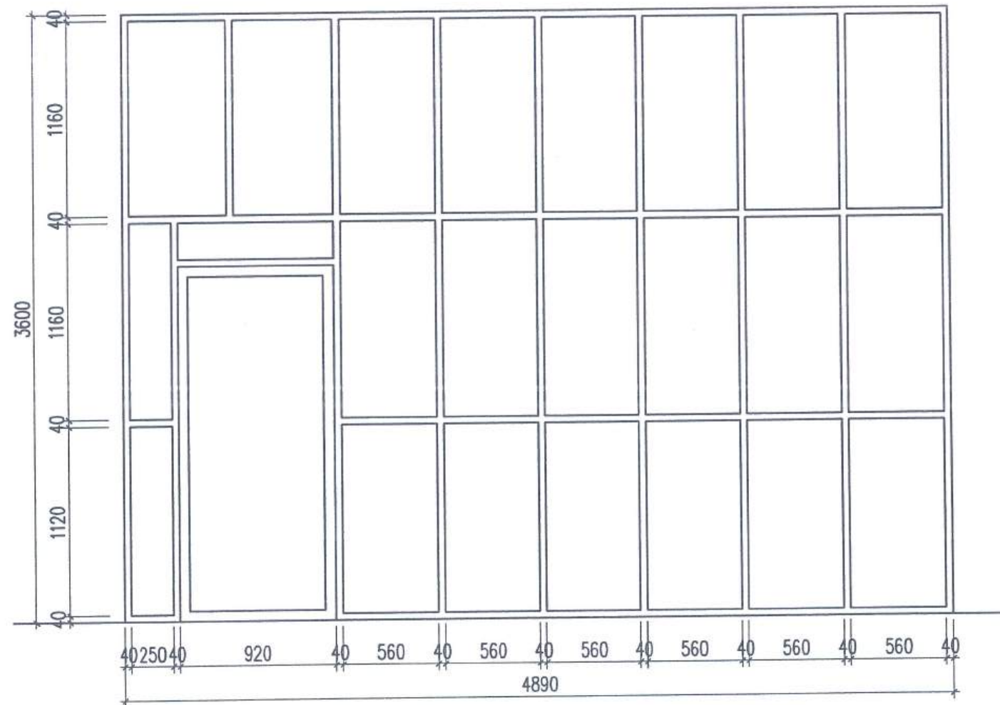
VÁCH THẠCH CAO
