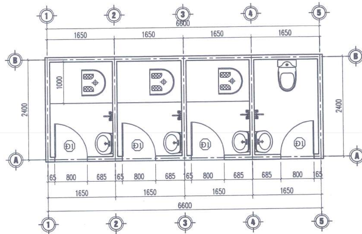
MẶT BẰNG
