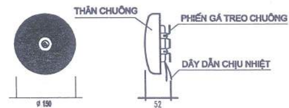
CHI TIẾT CHUÔNG BÁO CHÁY
