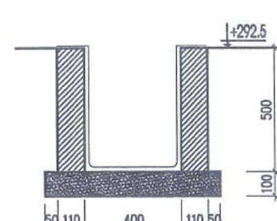
MẶT CẮT RÃNH HỖ H1-H2 TẠI H1
