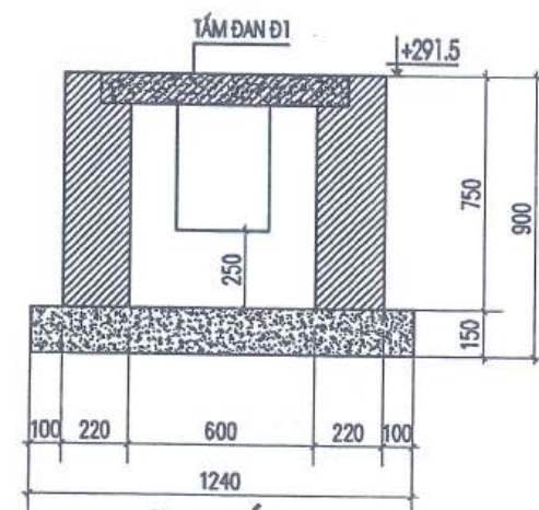
MẶT CẮT HỖ GA H3
