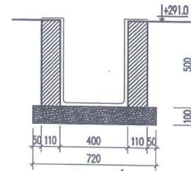
MẶT CẮT RÃNH HỖ H3-H4 TẠI H4
