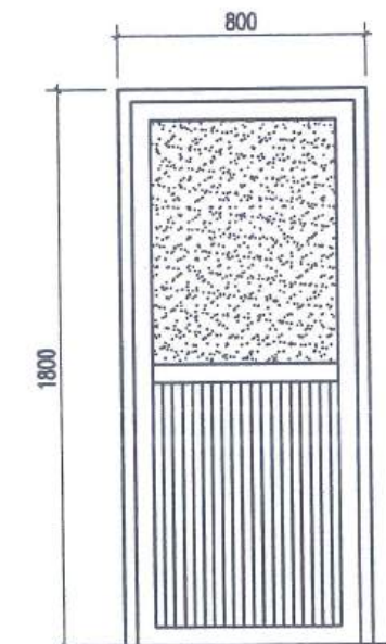
CỬA Đ1 (CỬA KÍNH KHUNG NHÔM, KÍNH DÁN 6.38MM)
