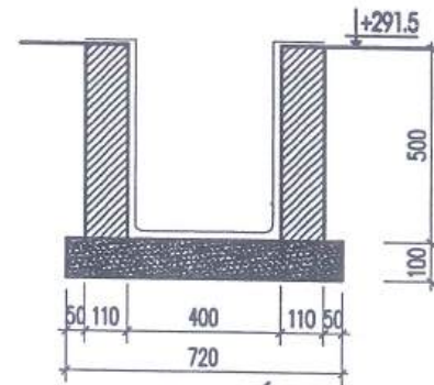
MẶT CẮT RÃNH HỖ H3-H4 TẠI H3
