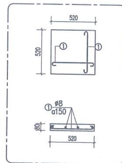
TẤM ĐAN Đ5 (SL= 01CÁI)
