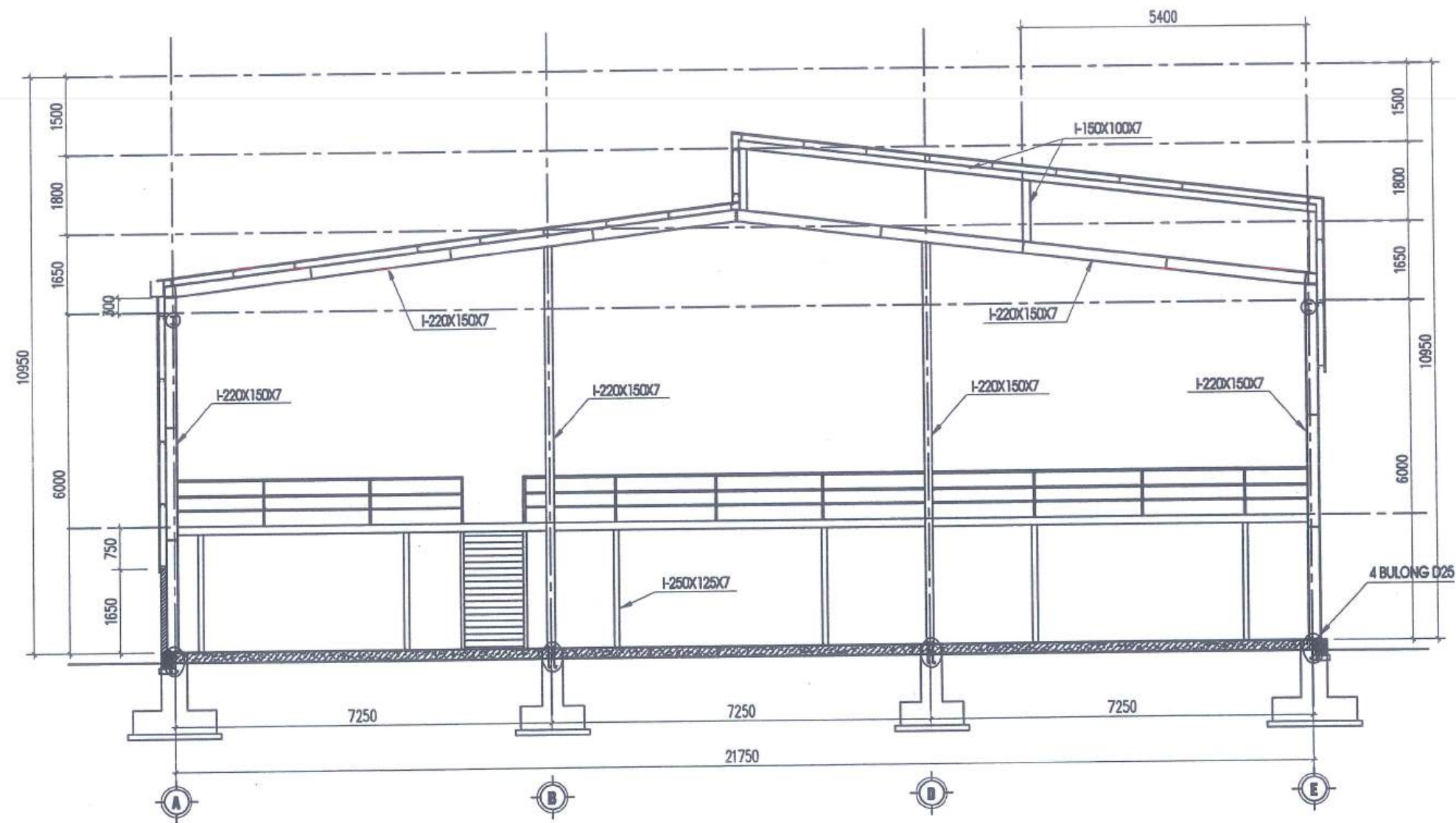
MẶT ĐÚNG KHUNG K2
