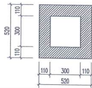
MẶT BẰNG HỐ THU H6
