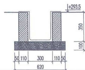
MẶT CẮT RÃNH HỖ R1-H1 TẠI R1
