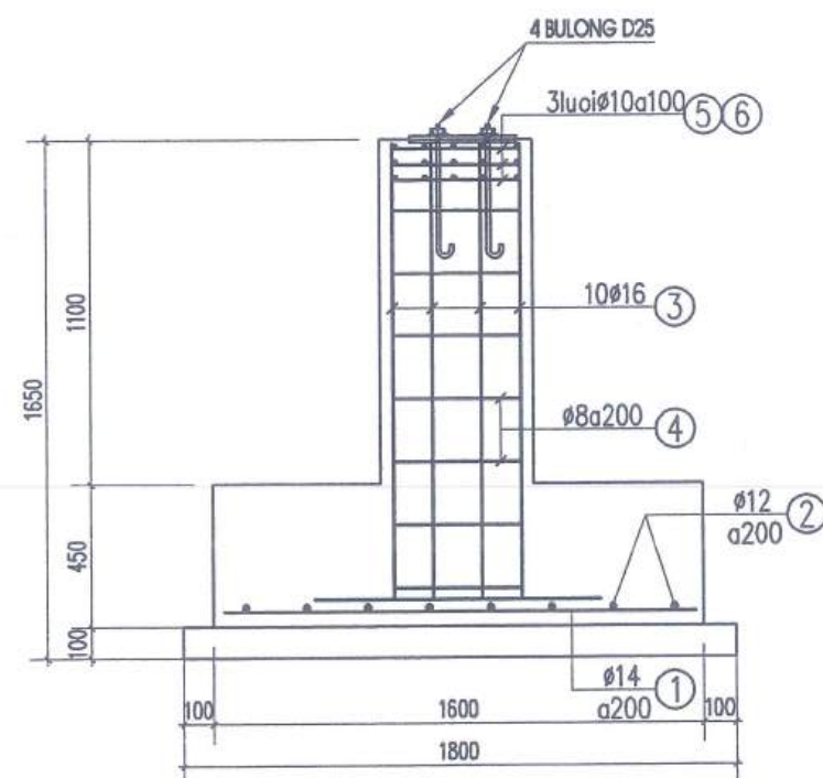
CẮT 1-1
