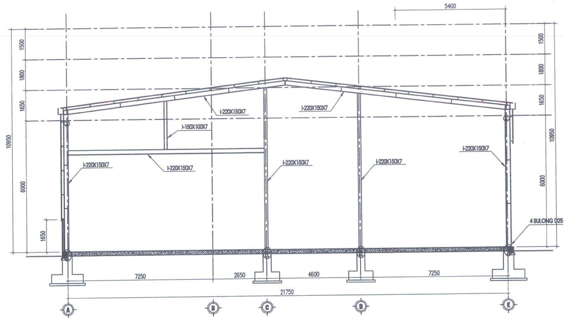
MẶT ĐÚNG KHUNG K2A
