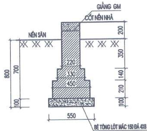
MÓNG MG-1
