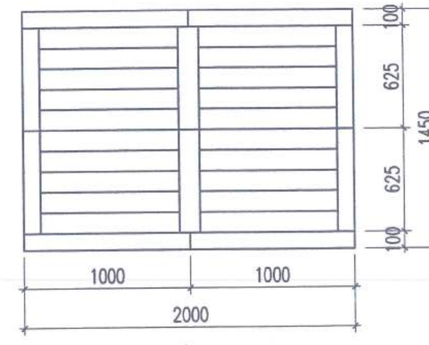
HOA SẮT CỬA S2
