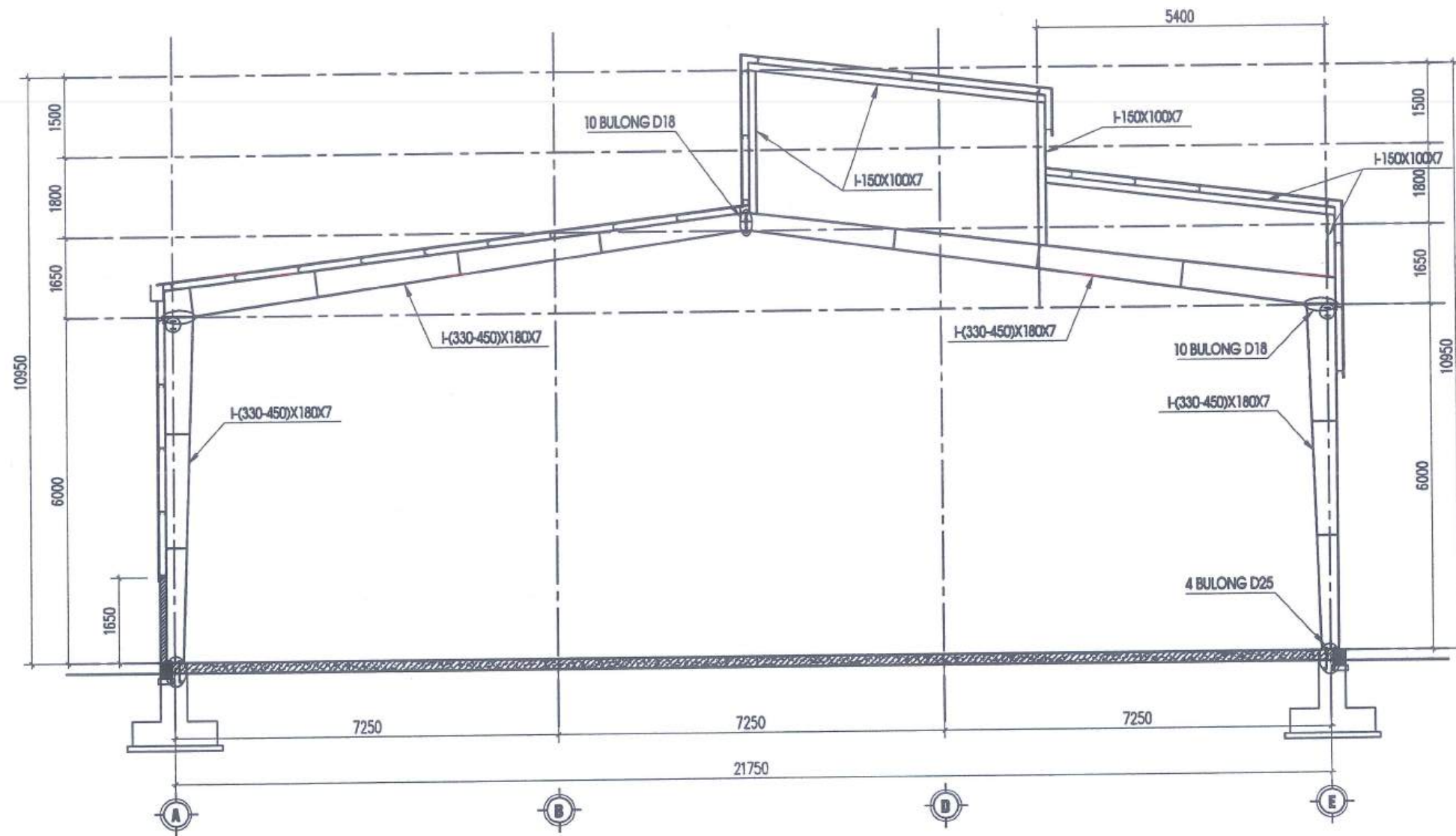
MẶT ĐỨNG KHUNG K1A
