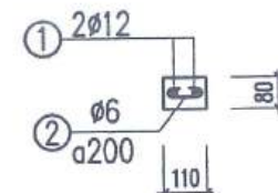
LANH TÔ
