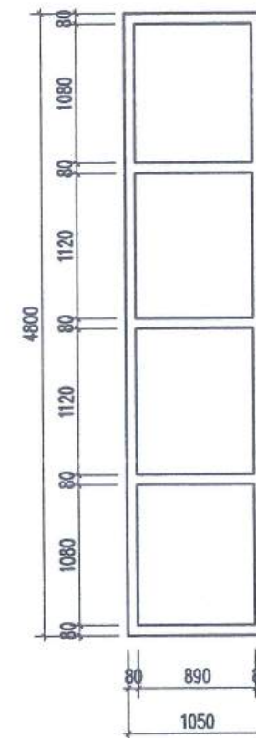
KHUNG CÁCH 1,05M (KHUNG SẮT HỘP 40X80X2)
