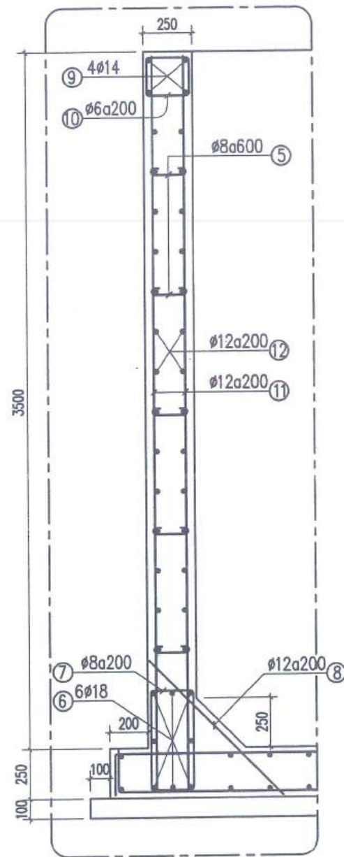
CẮT 1-1
