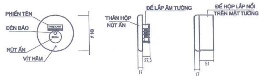
CHI TIẾT HỘP NÚTẤN BÁO CHÁY
