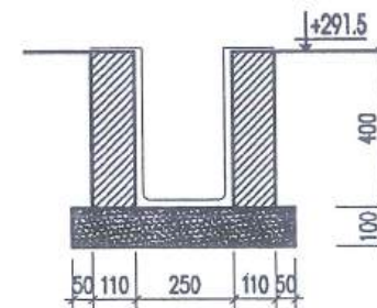
MẶT CẮT RÃNH HỖ R4-H3 TẠI H3
