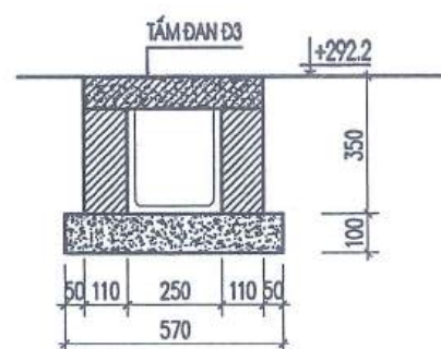
MẶT CẮT RÃNH KÍN R5-H4 TẠI R5
