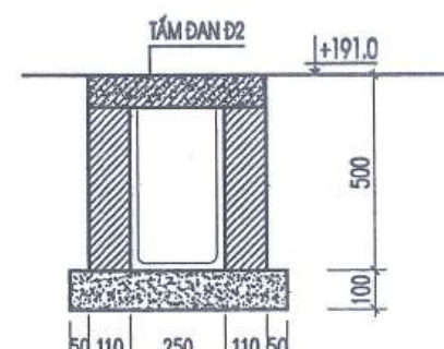
MẶT CẮT RÃNH KÍN R5-H4 TẠI H4
