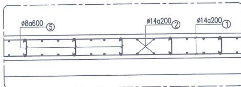
CỐT THÉP ĐÁY BỂ (ĐÁY CỐT 3.5M)
