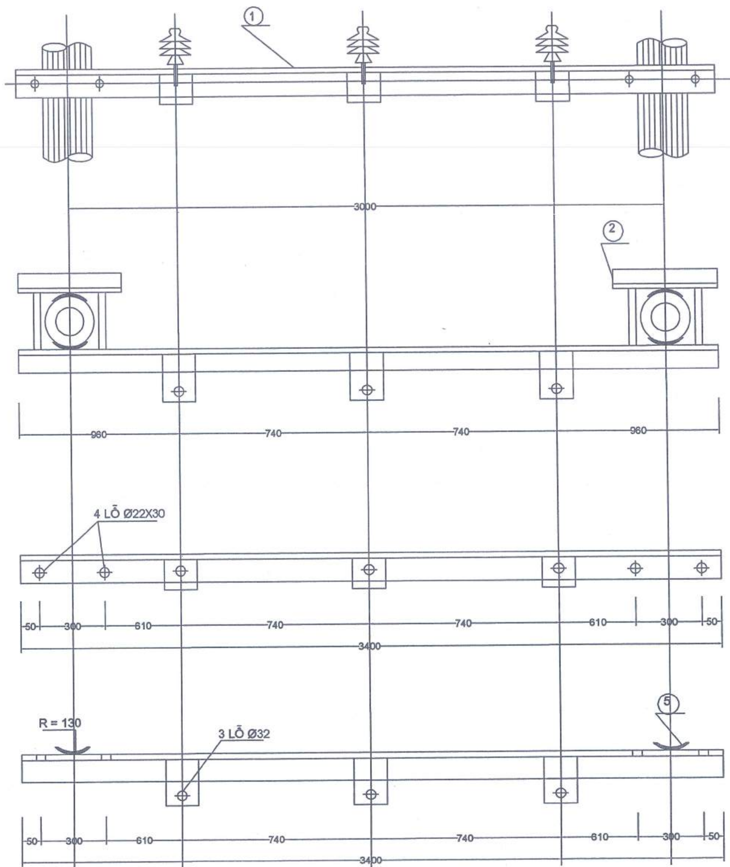
CHI TIẾT 1
