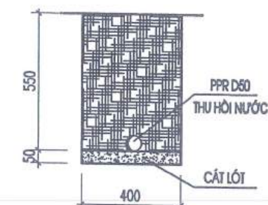
MẶT CẮT RĂNG ĐẶT ỐNG THU HỒI NƯỚC TÁI SỬ DỤNG
