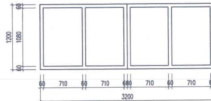
KHUNG CỬA SỔ (KHUNG THÉP HỘP 30X60X2)
