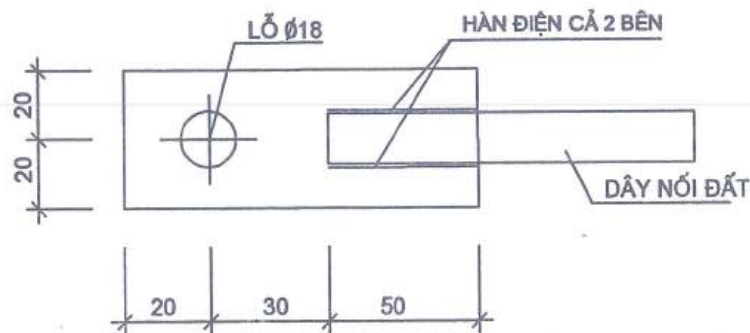
BẢN NỐI ĐẤT
