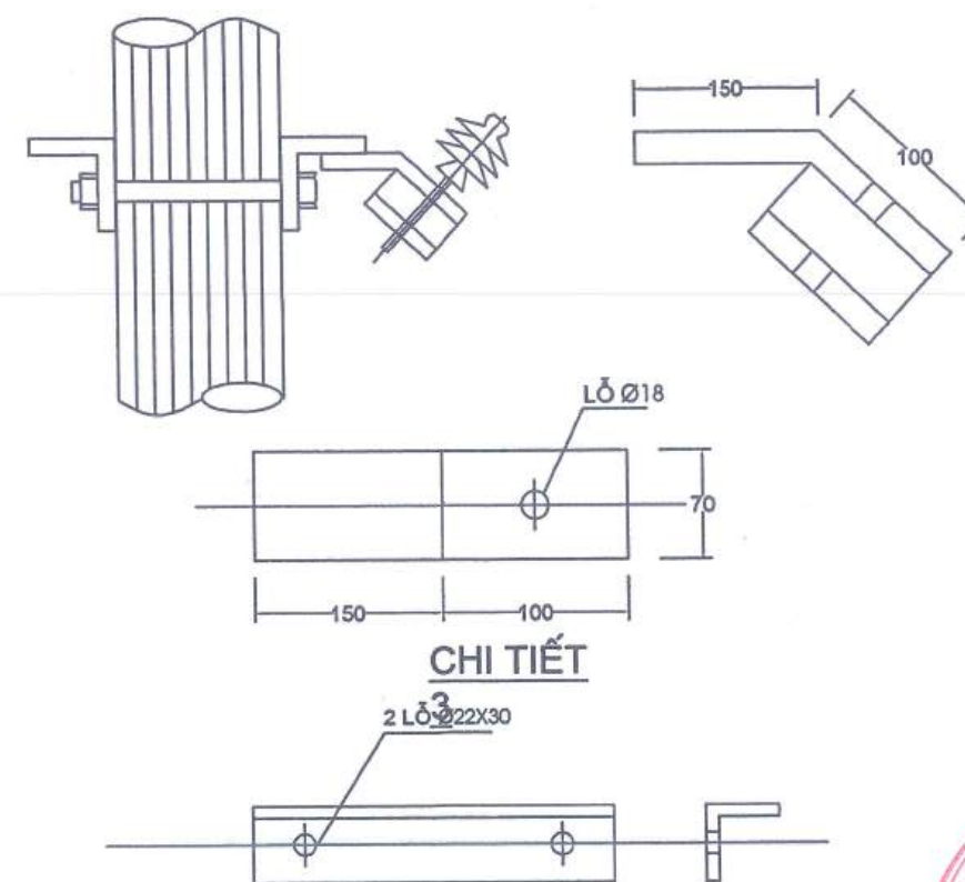
CHI TIẾT 2
