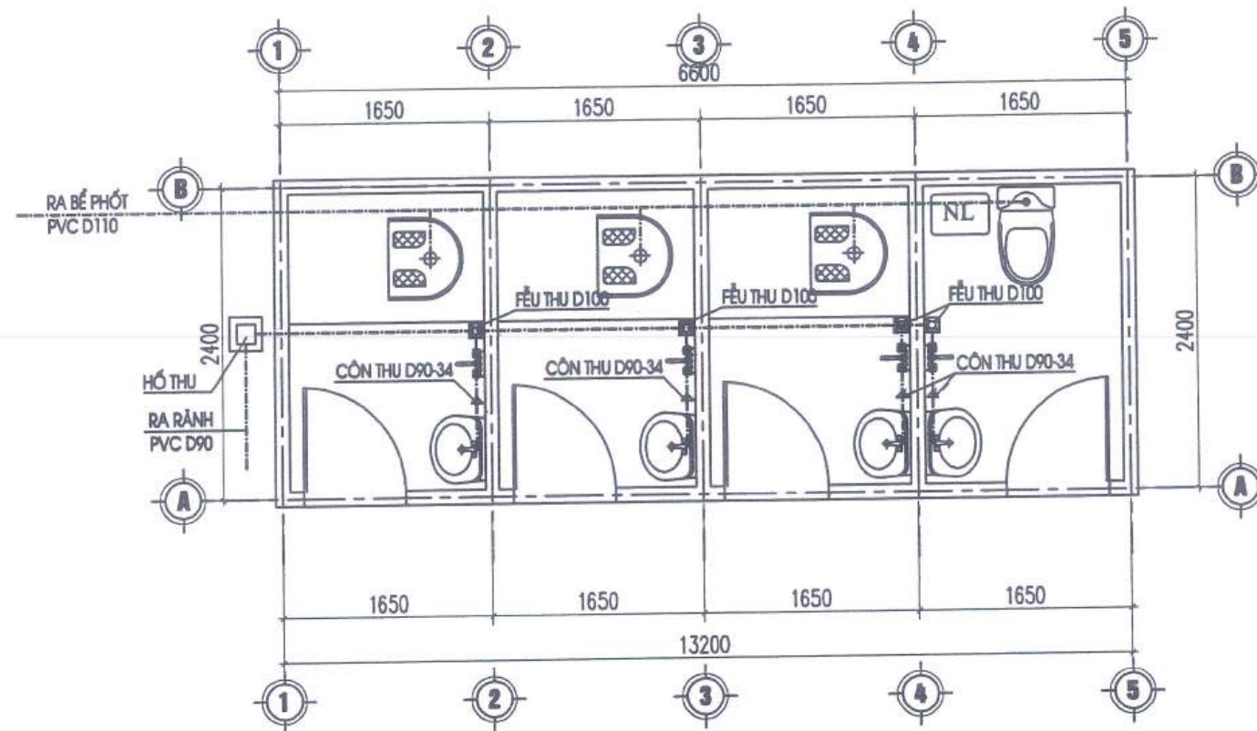
MẶT BẰNG THOÁT NƯỚC
