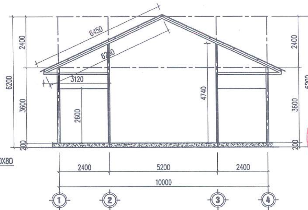
MẶT CẮT B-B
