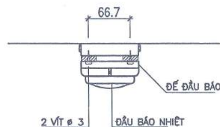
LẮP ĐẶT ĐẦU BÁO KHỎI QUANG HỌC DƯỚI DÂY TREO THÉP
