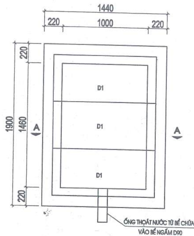
MẶT BẰNG HỒ TỰ NGẮM
