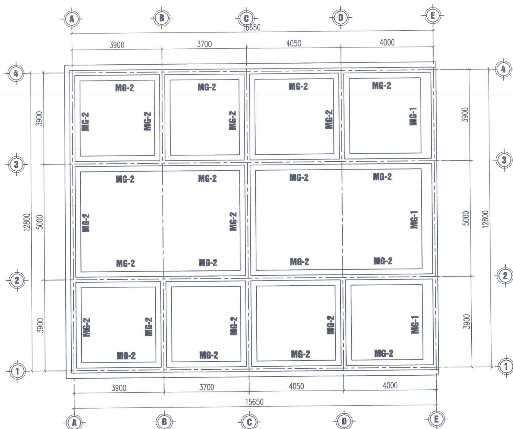
MẶT BẰNG MÓNG
