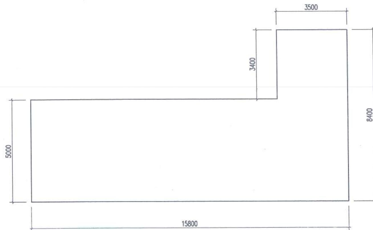
MẶT BẰNG (MÓNG BỐN CHỨA TÍNH DẦU)
