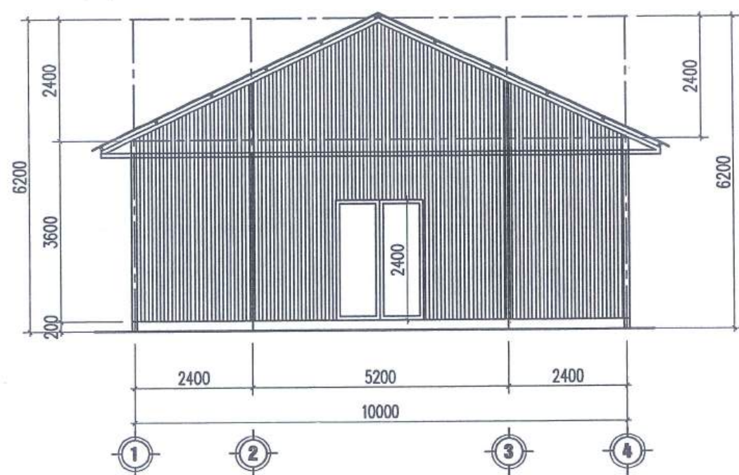
MẶT ĐÚNG
