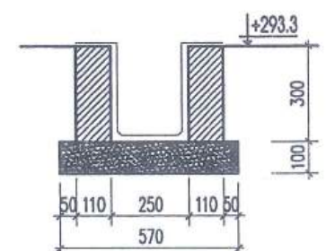
MẶT CẮT RÃNH HỖ R3-H2 TẠI R3
