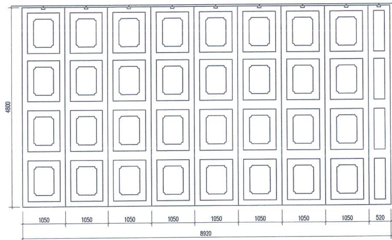
CỬA ĐI CHÍNH (CỬA KHUNG SẮT BỊT TÔN)
