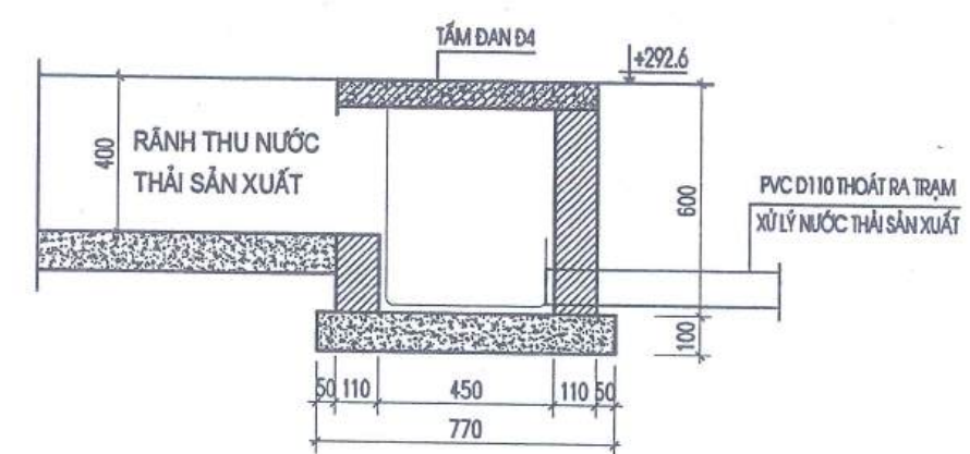
MẶT CẮT HỐ THU H7
