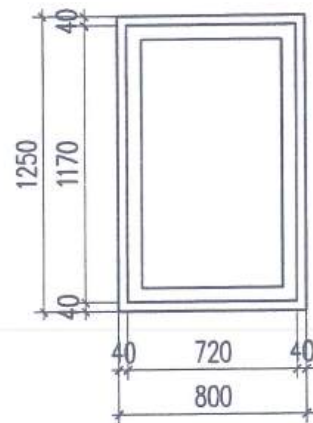
CỬA S1
