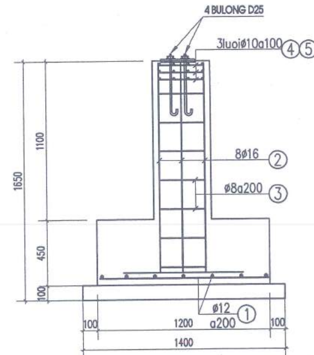
CẮT 2-2
