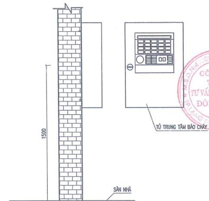
CHI TIẾT LẮP ĐẶT TỦ TRUNG TÂM BÁO CHÁY 5 KÊNH
