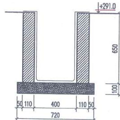
MẶT CẮT RÃNH HỖ H4-H5 TẠI H5
