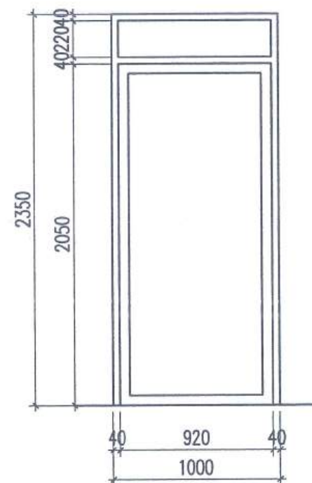
CỬA Đ2 (CỬA KÍNH KHUNG NHÔM, KÍNH DÁN 6,38MM)
