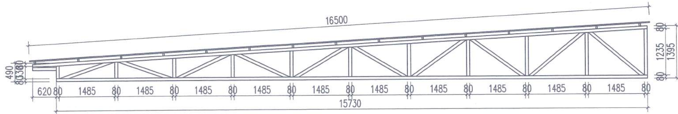
VÌ KÈO THÉP (THÉP HỘP 80X40 DÂY 1,4MM)
