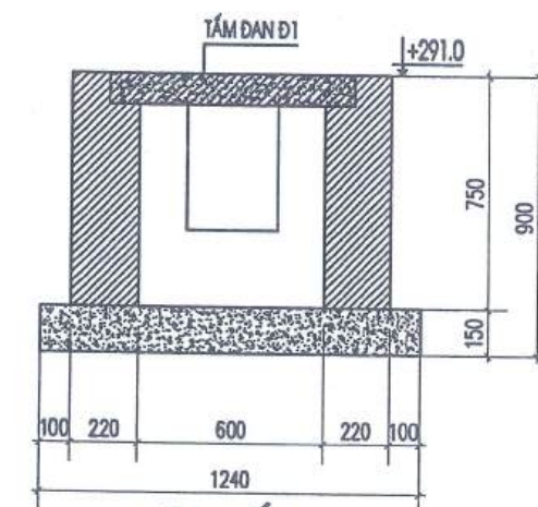
MẶT CẮT HỖ GA H4
