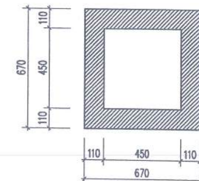
MẶT BẰNG HỐ THU H7
