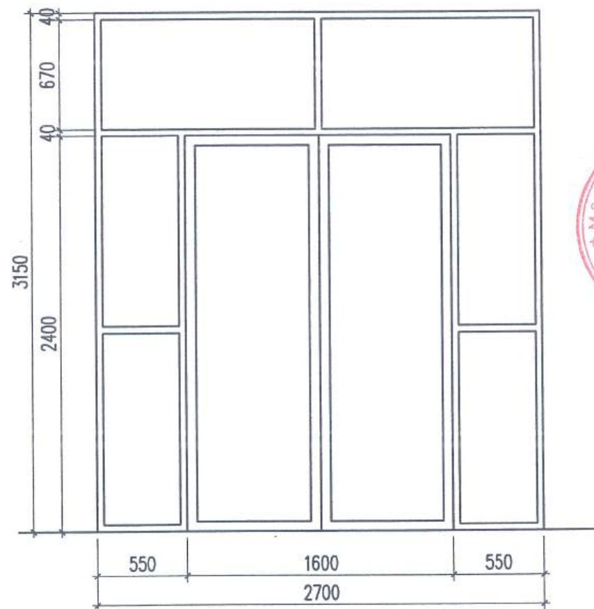
CỬA Đ3 (CỬA KÍNH KHUNG NHÔM, KÍNH DÁN 6,38MM)
