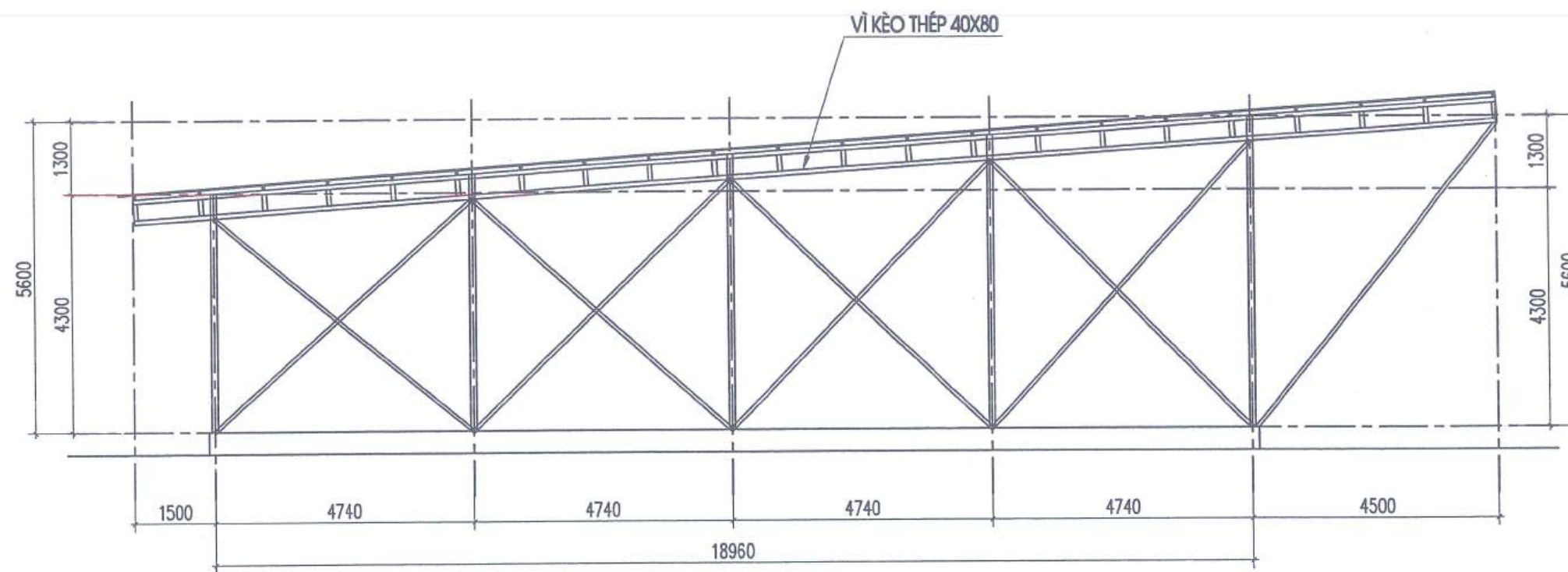
MẶT CẮT
