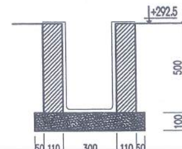
MẶT CẮT RÃNH HỖ R2-H1 TẠI H1
