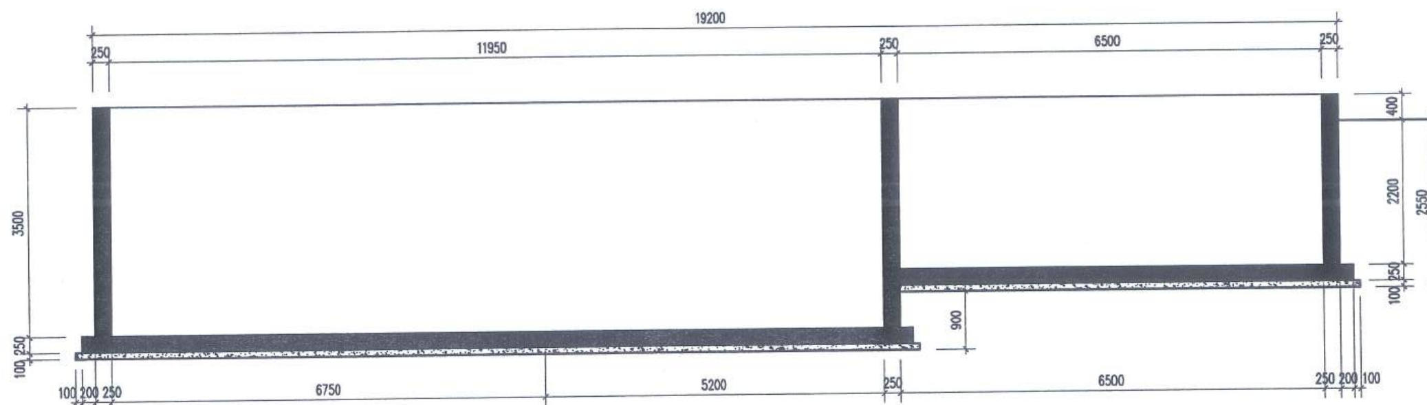
CẮT B-B
