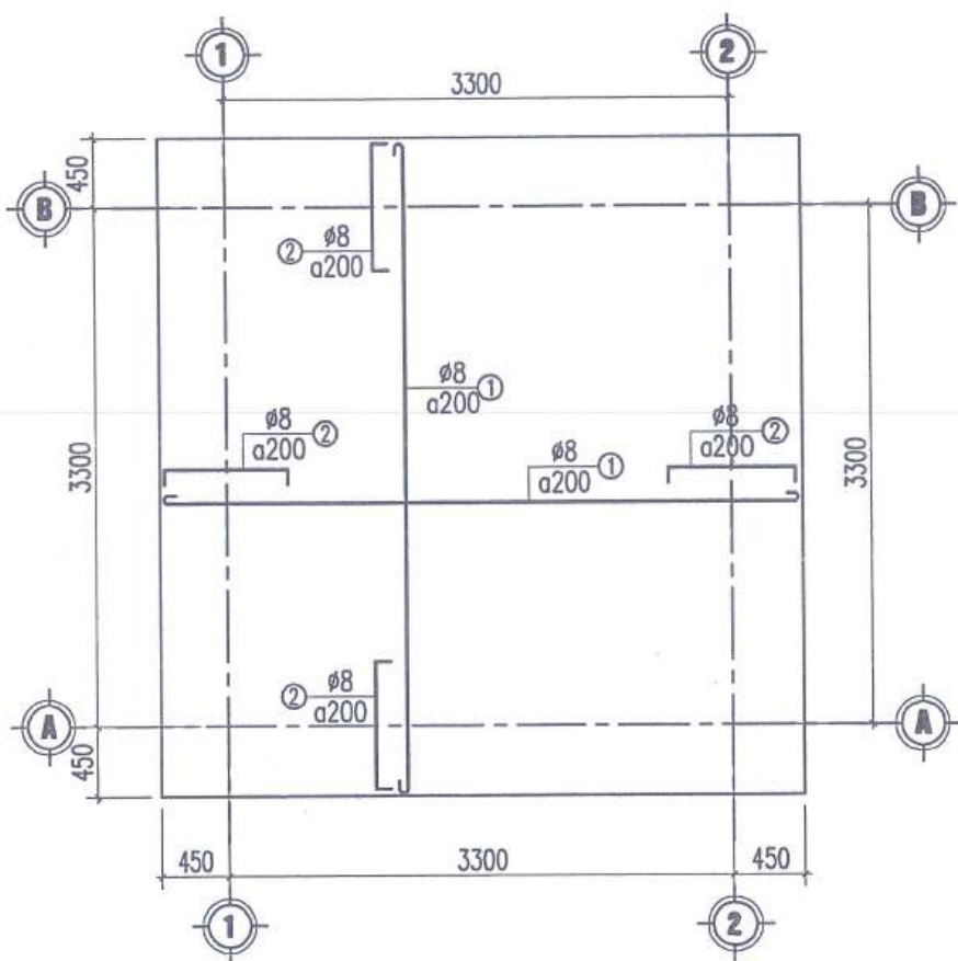
MẶT BẰNG CỐT THÉP MÁI
