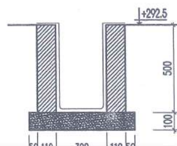
MẶT CẮT RÃNH HỖ R1-H1 TẠI H1
