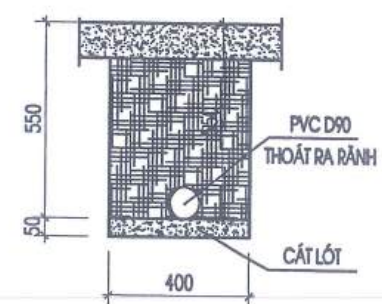
MẶT CẮT RĂNG ĐẶT ỐNG THOÁT NƯỚC THẢI SINH HOẠT
