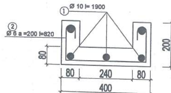
MĂNG THU NƯỚC
