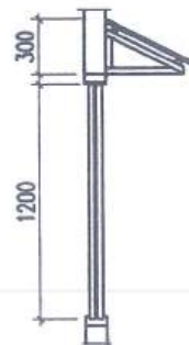
CẮT CỬA SỔ (CỬA KHUNG SẮT BỊT TÔN)
