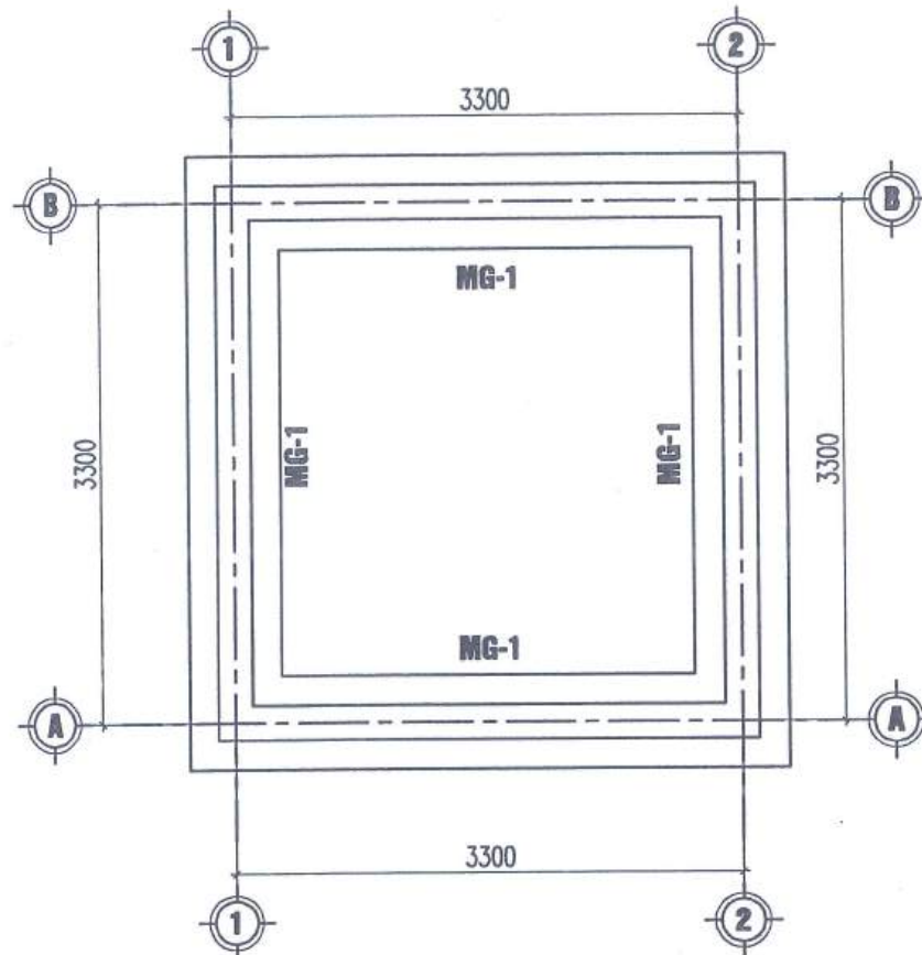
MẶT BẰNG MÓNG
