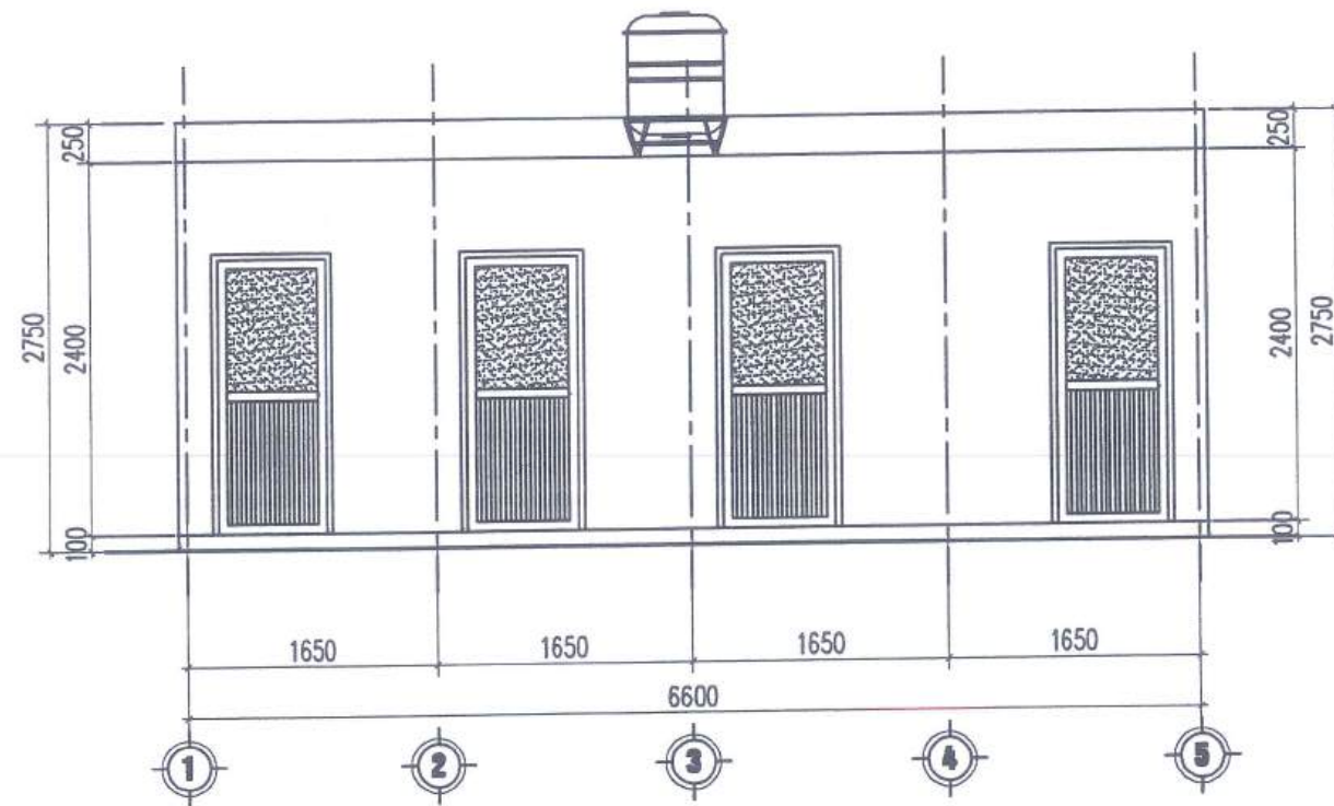
MẶT ĐỨNG TRỰC 1-5
