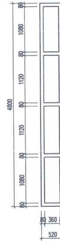
KHUNG CÁCH 0,52M (KHUNG SẮT HỘP 40X80X2)
