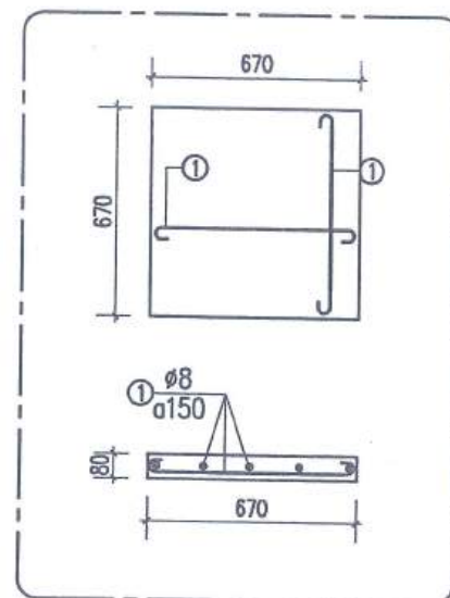
TẤM ĐAN Đ4 (SL= 01CÁI)
