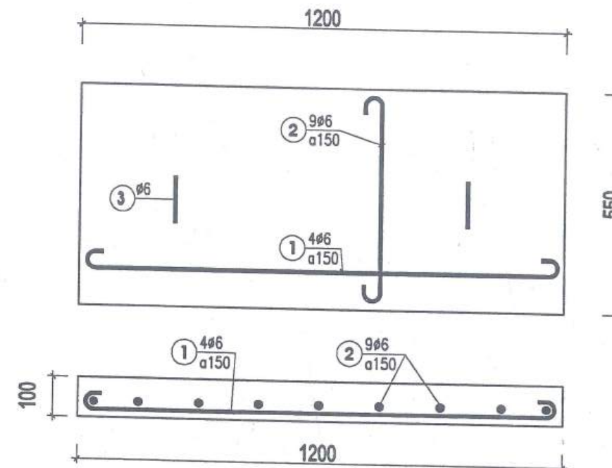
CHI TIẾT TẤM ĐAN D1 SL: 3 TẤM
