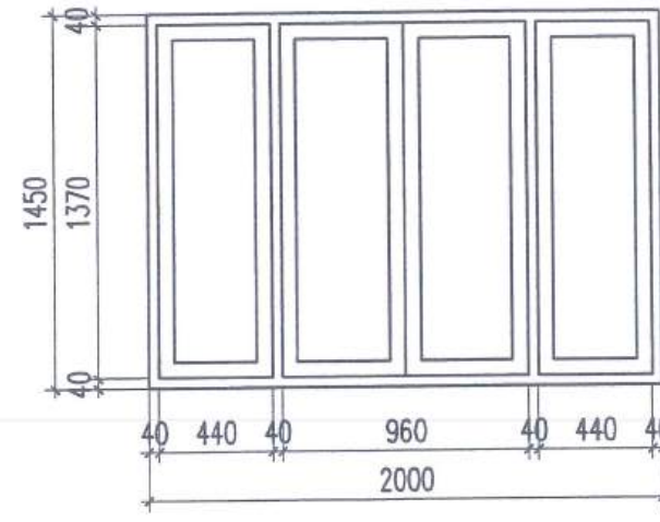
CỬA S2
