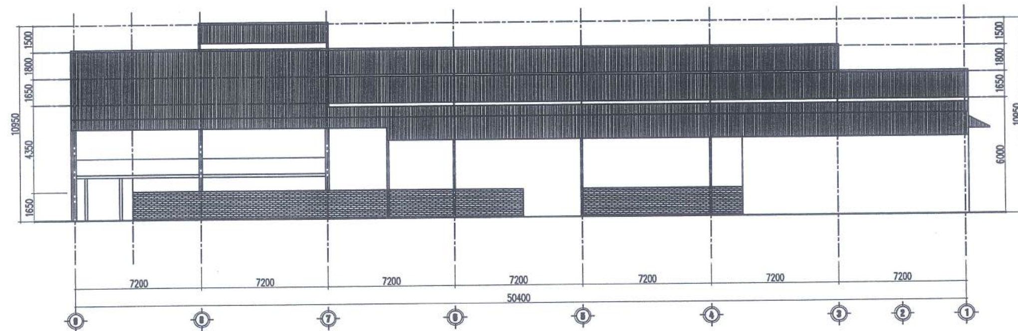
MẶT ĐỨNG TRỤC 9-1
