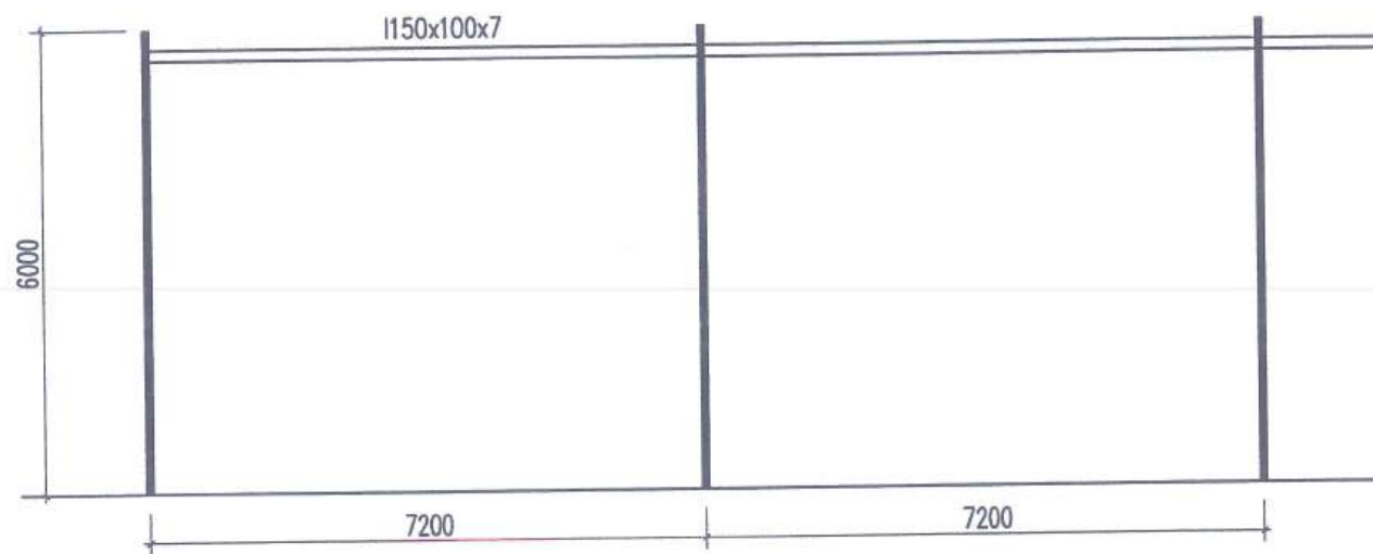
MÓNG ĐỨNG (GIẺNG ĐỈNH CỘT I150X100X7)
