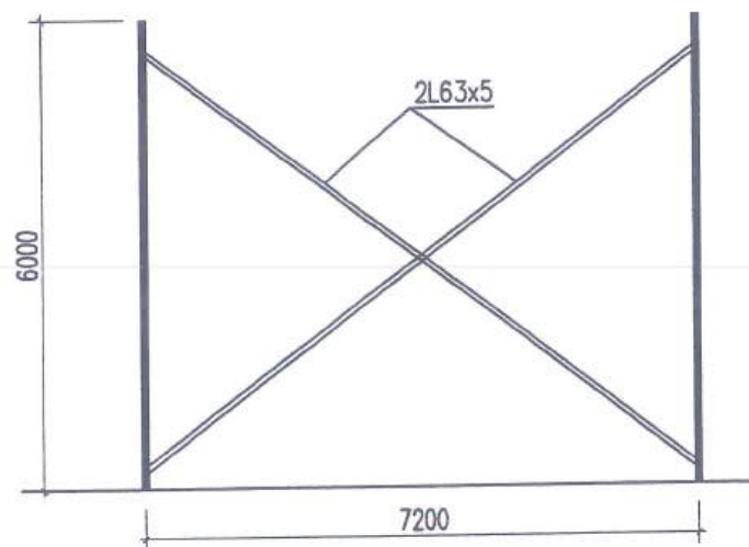
MÓNG ĐỨNG (GIẺNG KHUNG 2L63X5)
