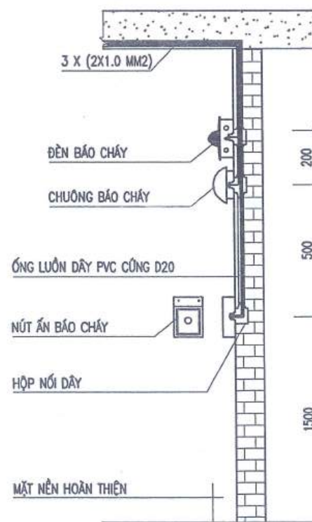
CHI TIẾT LẮP ĐẶT CHUÔNG, ĐÈN, NÚTẤN
