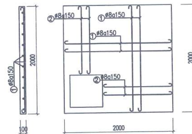
CỐT THÉP NẮP BỂ
