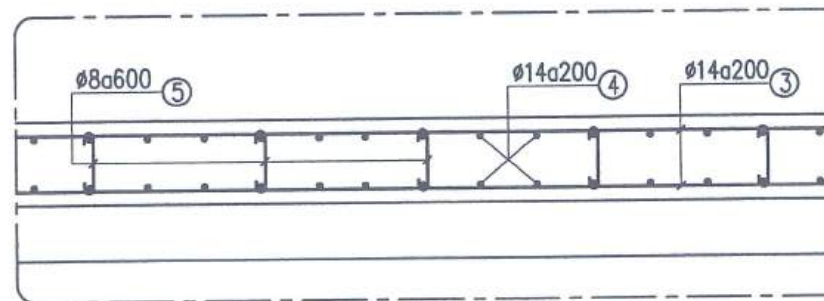
CỐT THÉP ĐÁY BỂ (ĐÁY CỐT 2.6M)
