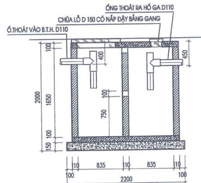
MẶT CẮT 1-1
