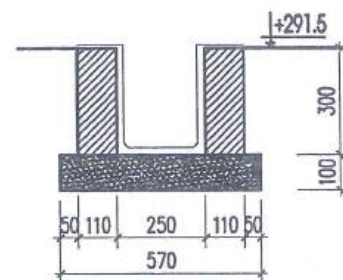
MẶT CẮT RÃNH HỖ R4-H3 TẠI R4
