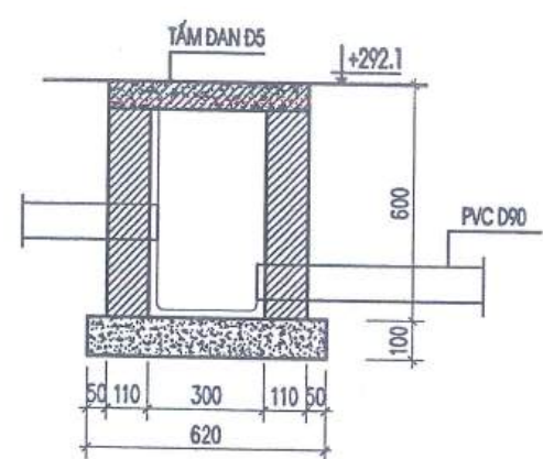
MẶT CẮT HỐ THU H6
