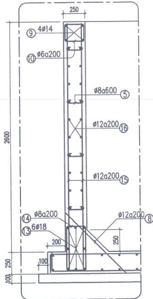
CẮT 2-2
